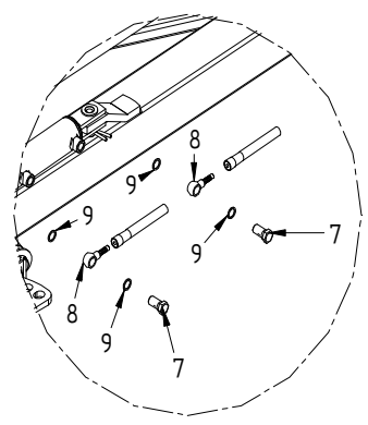
DETTAGLIO A
